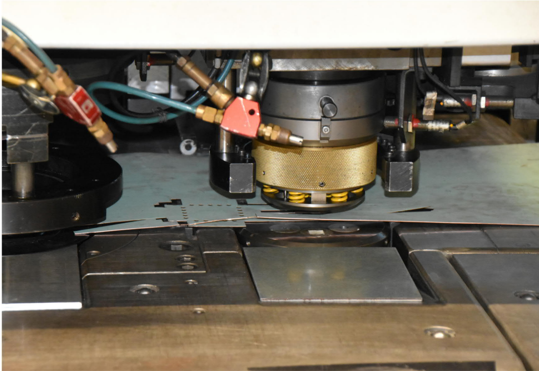
Der Stanzvorgang
